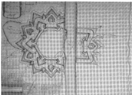
Storff's ontwerp voor de vernieuwing van de vesting Grave uit 1679. Het linkse deel - de wal om de stad - is uitgevoerd, het rechte deel - het bruggehoofd over de Maas - niet. Aanwezig in Det Kongelige Bibliotek, Kopenhagen.
