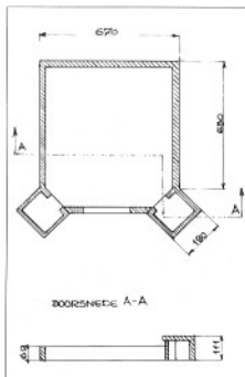
Plattegrond en doorsnede van een geschutsofstelling.
