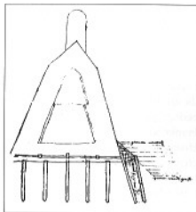
De schets van de 'Amsterdamse beer' van juli 1678. Rechts worden de waterstand en de bodem van de gracht aangegeven. Het houten fundament stond als een heuvel in de gracht. Door het aanbrengen van een kleipakket werd het mankement provisorisch gerepareerd.
